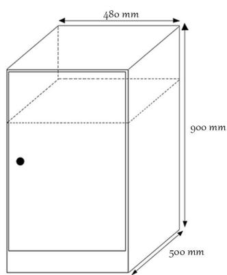
MUEBLE DE UNA PUERTA
