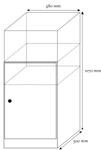
MUEBLE DE UNA PUERTA
